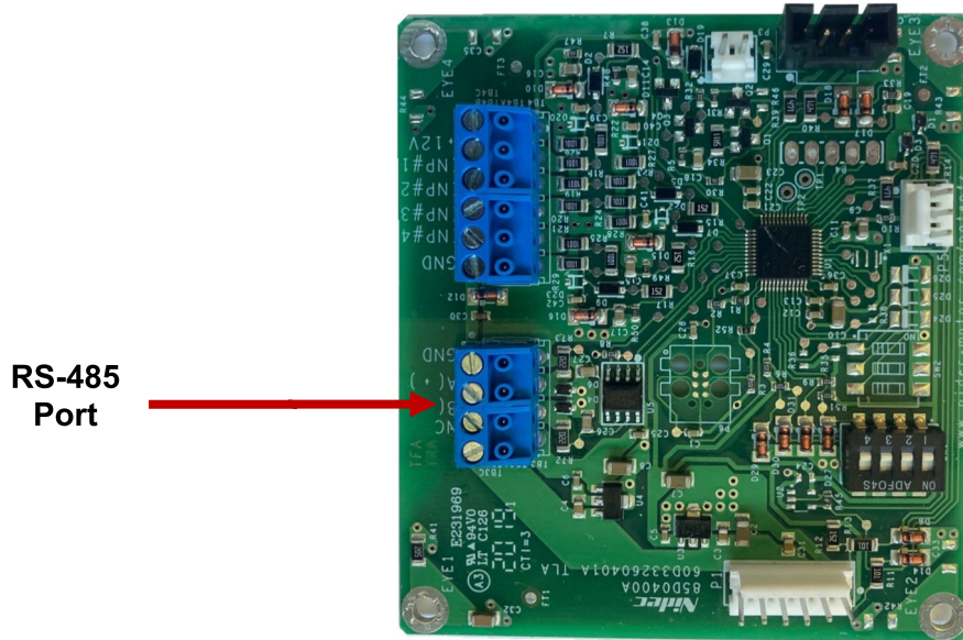
RS-485 Port on the DI Board
